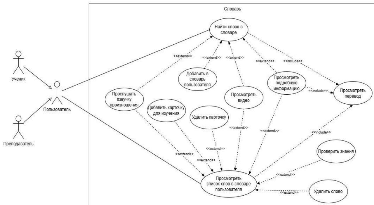
Рисунок 2. Диаграмма Use Case для версии 2.0 веб-приложения Chatty
